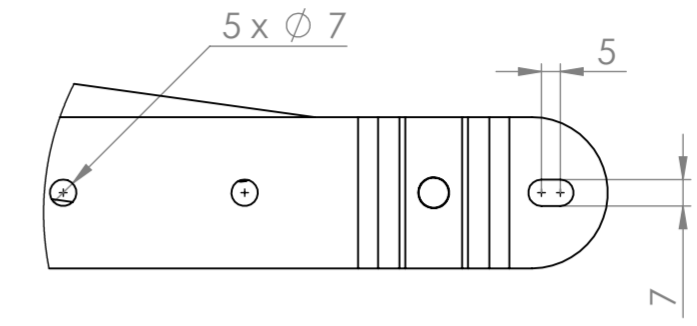
SZCZEGÓŁ A SKALA 1:2
