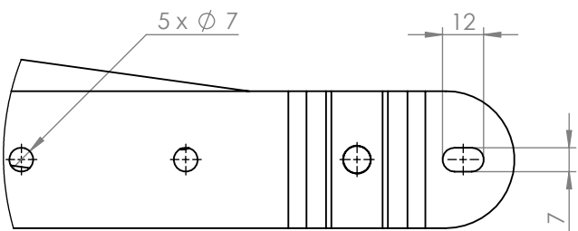
SZCZEGÓŁ D SKALA 1 : 2
